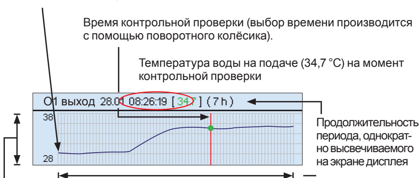
О1 График температуры воды на подаче
